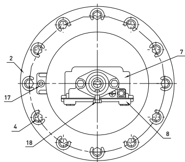
Вигляд зверху
